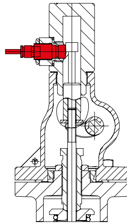
Näherungsschalter
