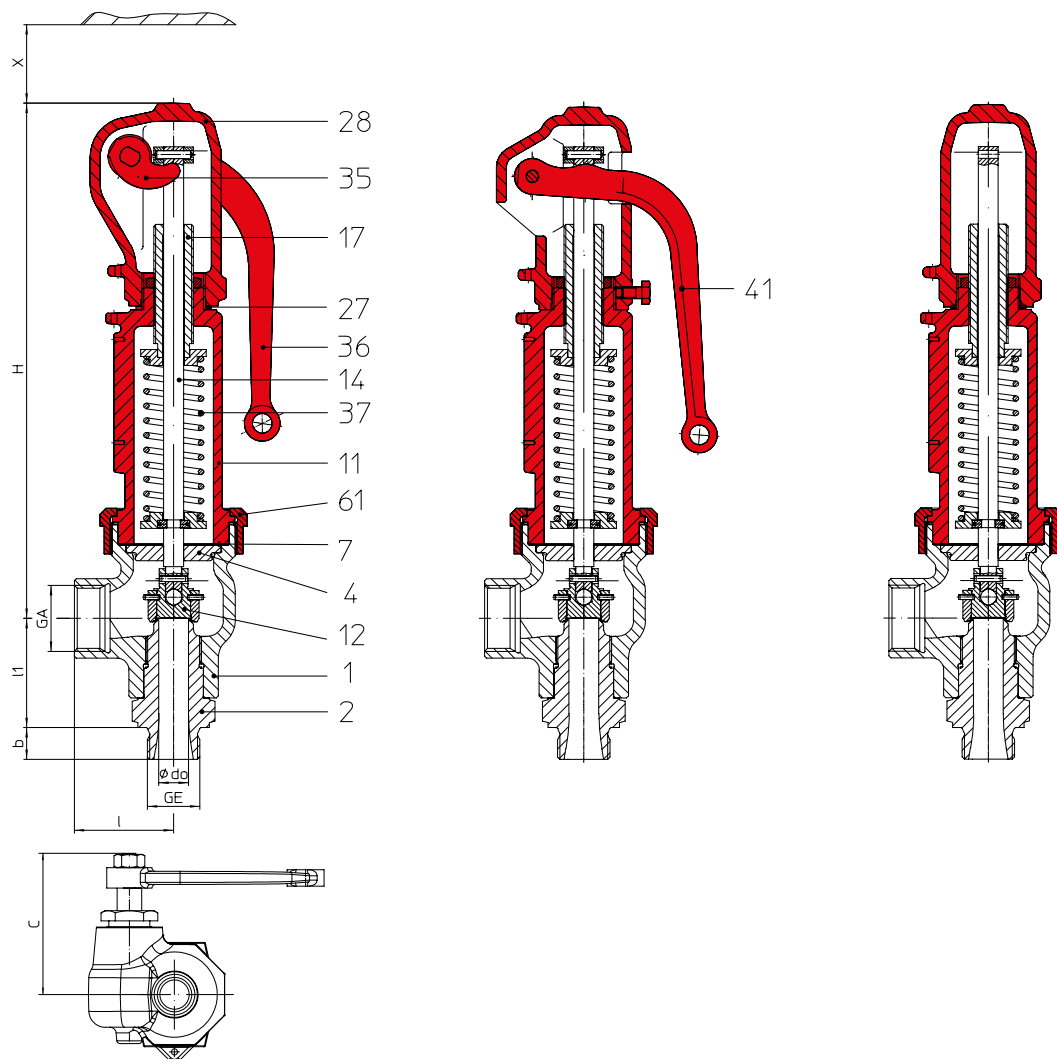
Серия ... 941 закрытый рычаг подрыва, закрытая крышка
