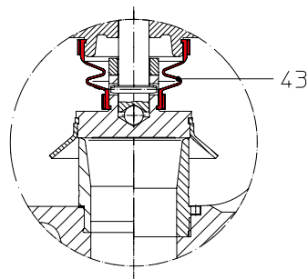
(Конструкция DN 20-100) (Конструкция DN125-150) Золотник с металлическим уплотнением, сиффон из EPDM
