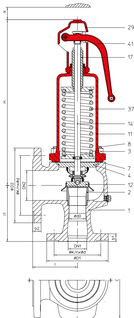
Серия ... 904 открытый рычаг подрыва, закрытая крышка
