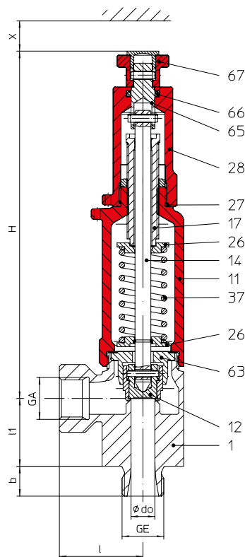
Серия ...951 закрытая кнопка подрыва
