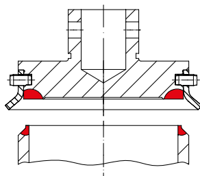
Седло 1.4571 / стеллит No. 21 Золотник 1.4571 / стеллит No 6 Седло SA479Gr.316Ti / стеллит No. 21 (SAFE-SN ANSI) Золотник SA479Gr.316Ti / стеллит No. 6 (SAFE-SN ANSI) съёмная оснастка для подрыва
