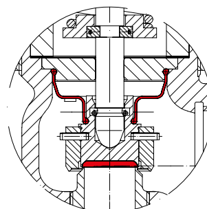
Fig. ... 945 Clapet avec insert en EPDM; Soufflet en EPDM
