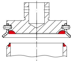
Siège 1.4571 / Stellite n° 21 Clapet 1.4571 / Stellite n° 6 Siège SA479Gr.316Ti / Stellite n° 21 (SAFE-SN ANSI) Clapet SA479Gr.316Ti / Stellite n° 6 (SAFE-SN ANSI) déflecteur de clapet amovible
