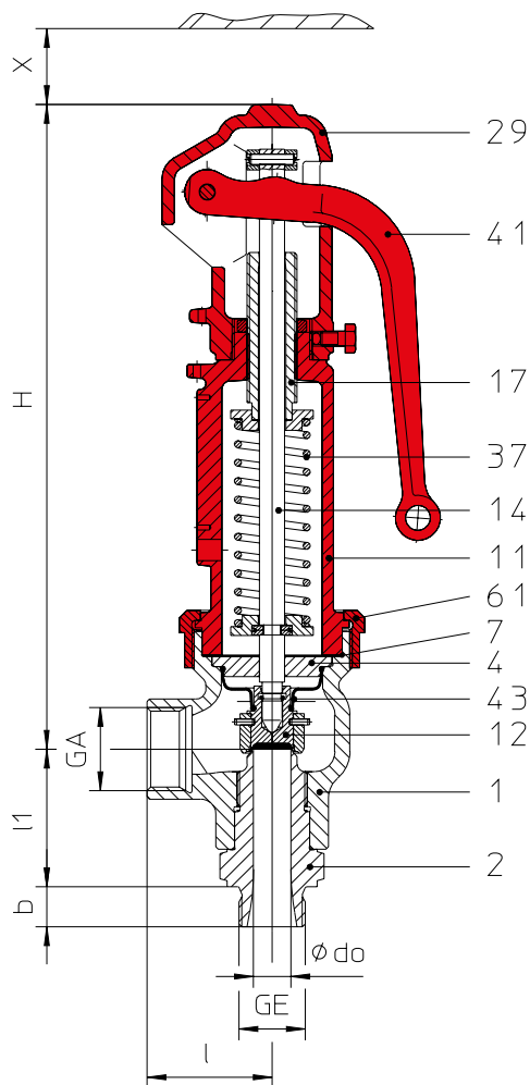
Fig. ... 945 bouchon de levier ouvert, chapeau fermé
