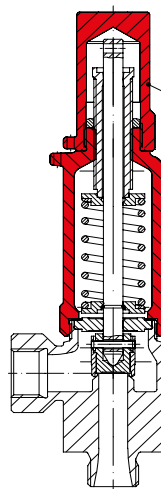
Fig. ... 963 bouchon étanche aux gaz
