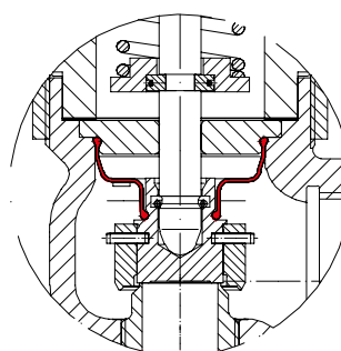
Fig. ... 946 Clapet à portée métallique. Soufflet d'étanchéité en EPDM
