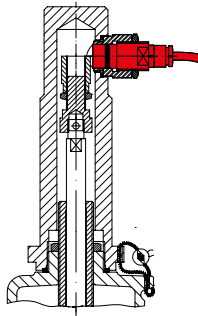
Nährungsschalter
