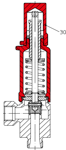
Fig. ... 963 gasdichte Kappe
