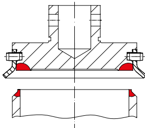
Sitz 1.4571 / Stellite No. 21 Kegel 1.4571 / Stellite No. 6 Sitz SA479Gr.316Ti / Stellite No. 21 (SAFE-SN ANSI) Kegel SA479Gr.316Ti / Stellite No. 6 (SAFE-SN ANSI) lösbare Hubhilfe
