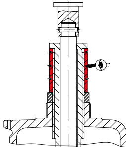
Sperrhülse
