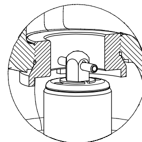
Clapet DN 40 - 150
