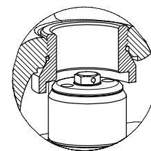
Clapet DN 15 - 32
