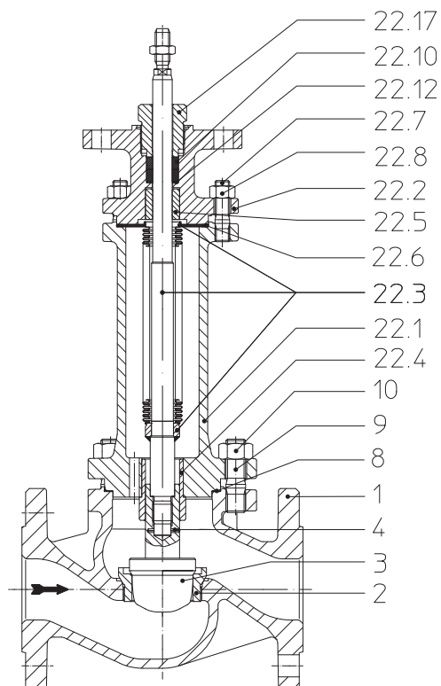
Рис. 2: BR 471 DN15-150
