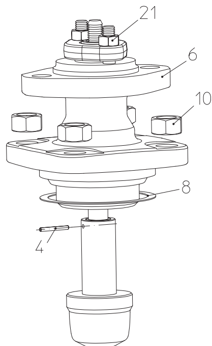
Рис. 16: BR 470
