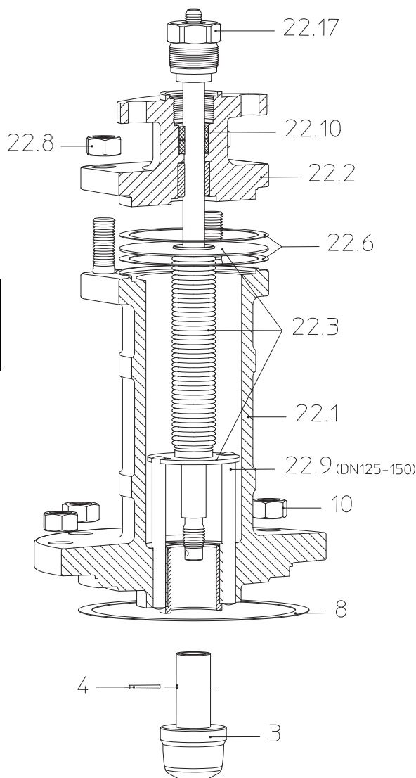
Рис. 14: BR 471 DN 15-150
