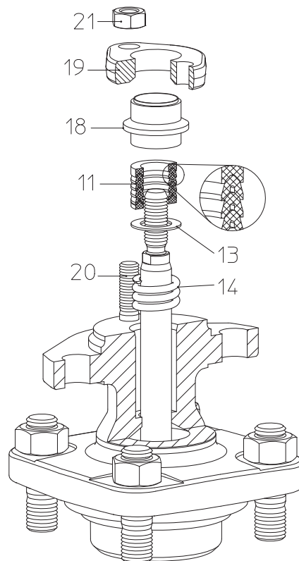
Рис. 10: сальниковые кольца DN15-150
