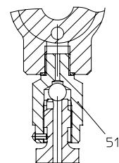
Сливной клапан
