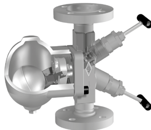
CONA®SC All-in-one (Изображено с опциональным продувочным клапаном)
