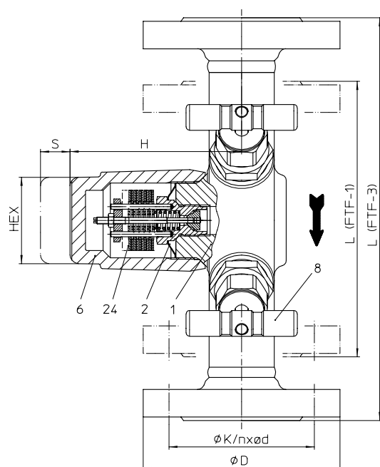
Серия 60А....1 с фланцами (приток справа)
