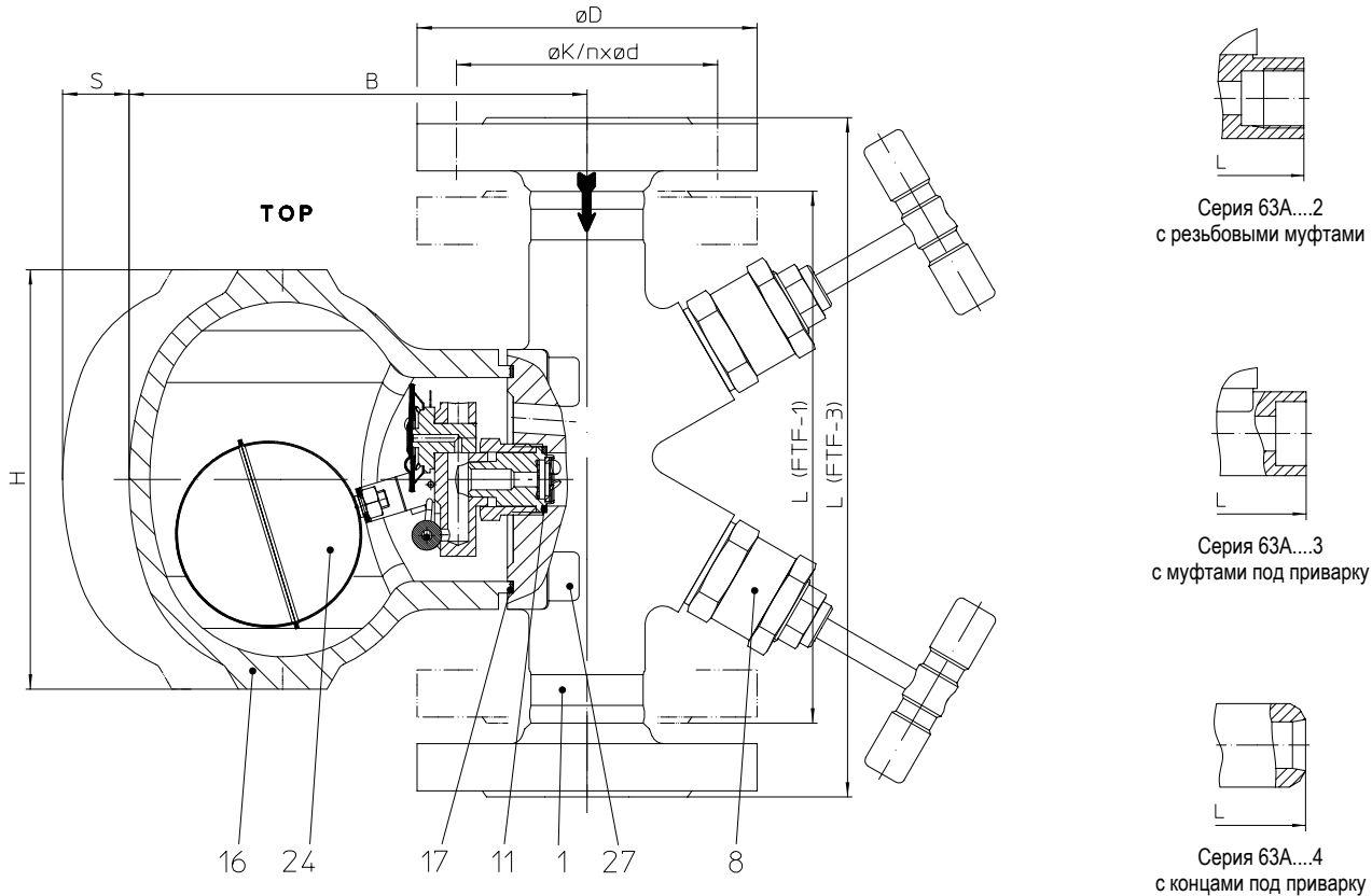
Серия 63A....1 с фланцами (приток сверху )
